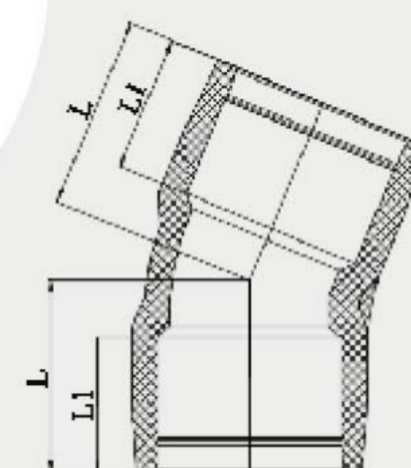
CODO 22.5°
