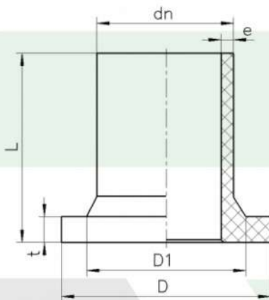
Accesorios Termofusión HDPE Stub end SDR11
